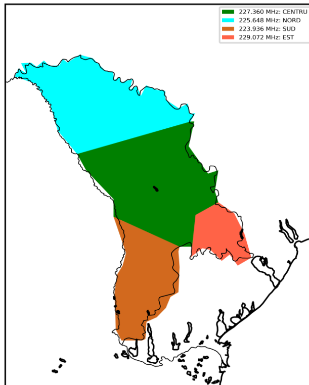
Configuratie alocari MUX DAB+ B
