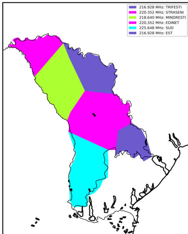
Configuratie alocari MUX DAB+ A
